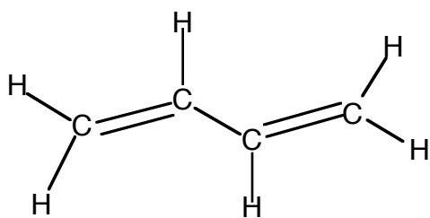
1,3-butadiene
